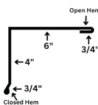
SS200 Rake
